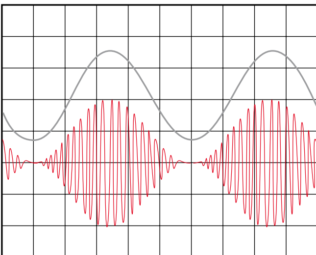
Externe Quelle: U_e = 1,40 V_p , 1 kHz, 1 V/div; HM8131-2: U_a = 10 V_{\text{pp}} , 20 kHz, 5 V/div ; 100% Modulation am Generator eingestellt
