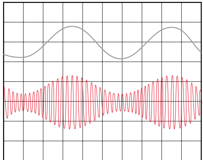
Generator1: U_e = 0,70 V_p , 1 kHz, 1 V/div; HM8131-2: U_a = 10 V_{\text{pp}} , 20 kHz, 5 V/div; 100% Modulation am Generator eingestellt → nur 50% Modulation
