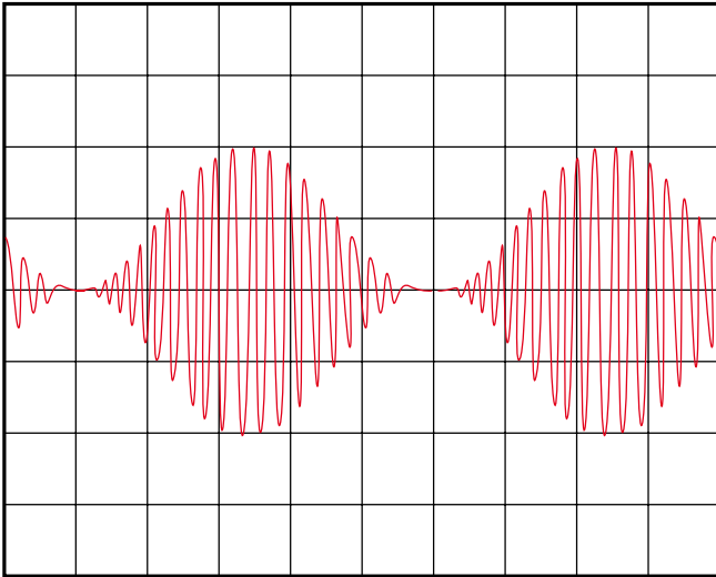
Interne Signalquelle, HM8131-2: U_a = 10 V_{\text{pp}} , 20 kHz, 5 V/cm 100% Modulation am Generator eingestellt
